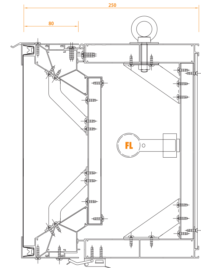
SK-250F 施工例
