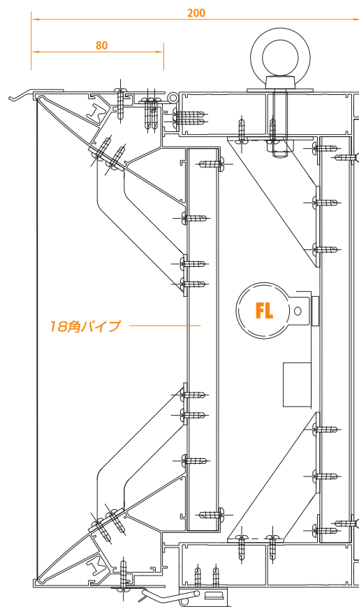
SK-200F 施工例
