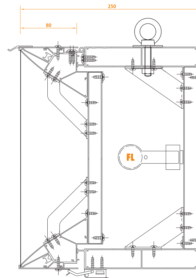
SK-80F (両面仕様) 施工例
