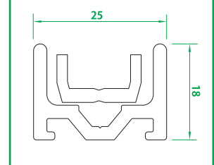
SK展張レール18
